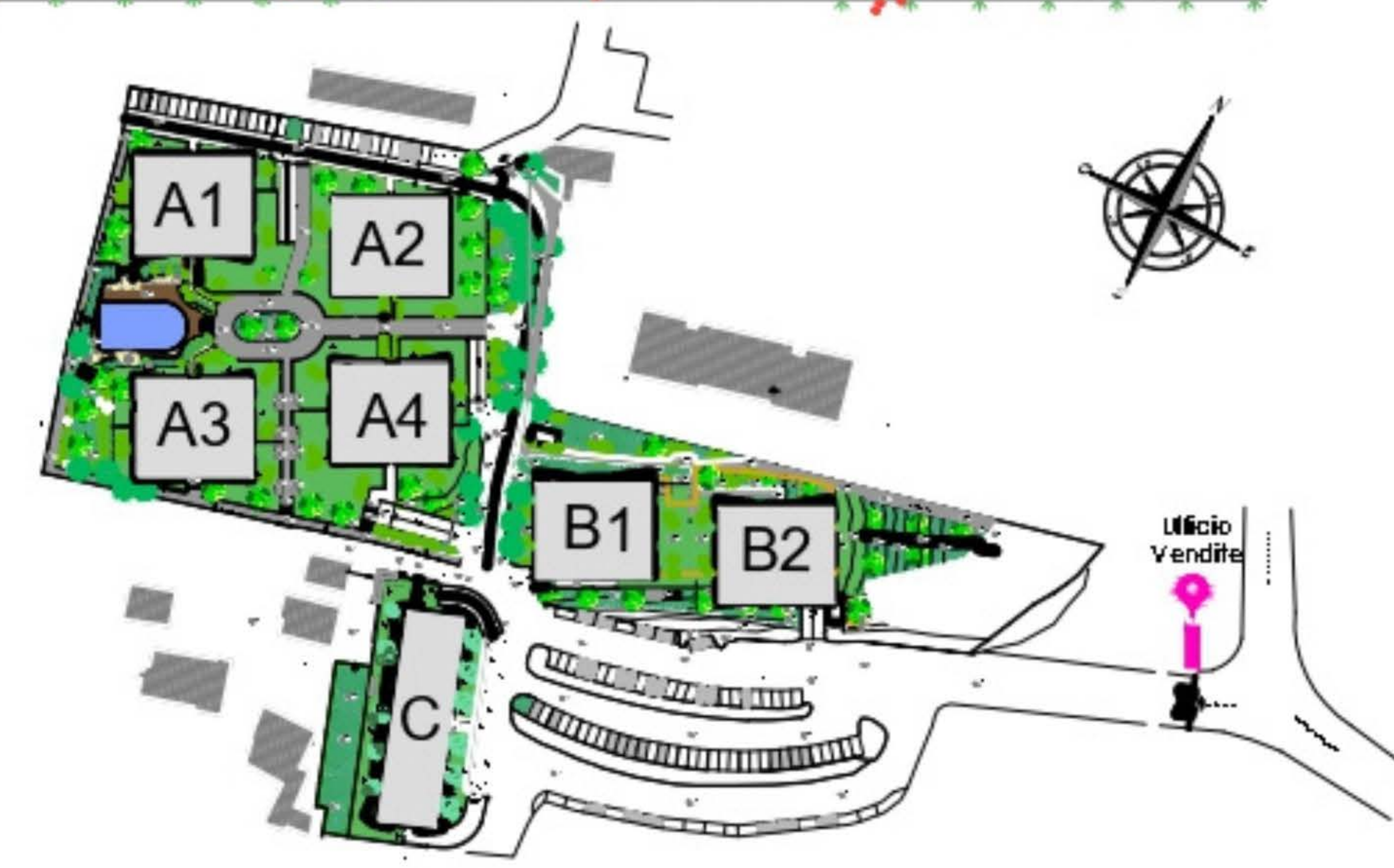
PLANIMETRIA GENERALE
